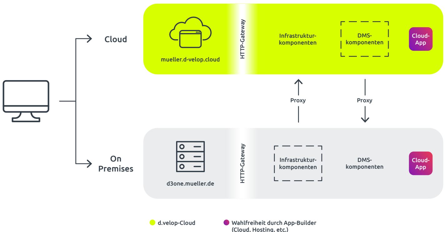
Schematische Darstellung von d.velop documents im Hybridbetrieb
